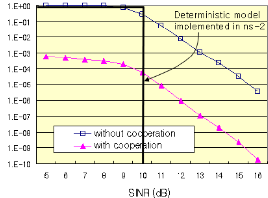
(b) FER versus SINR
